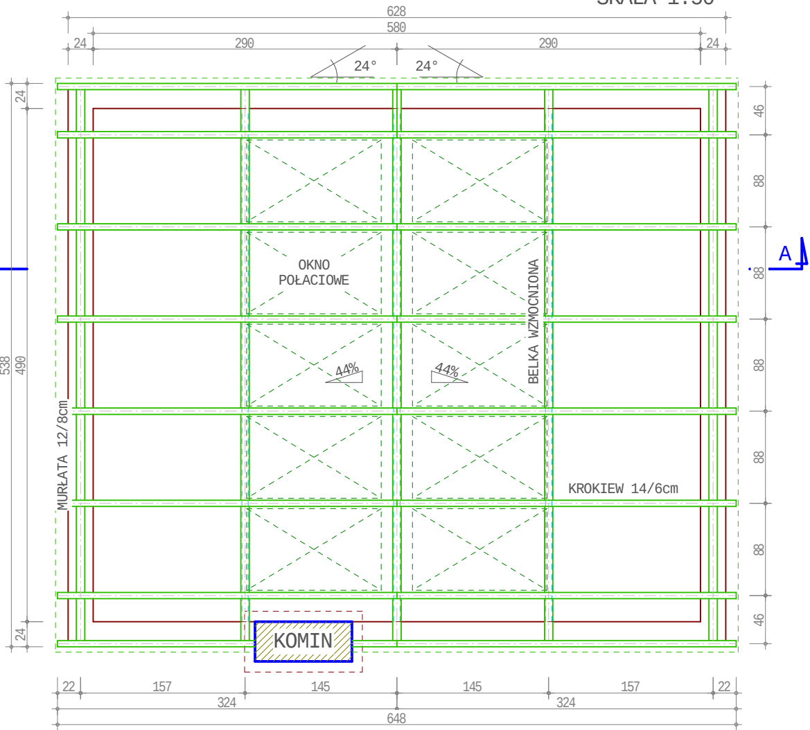
RZUT SKALA 1:50
